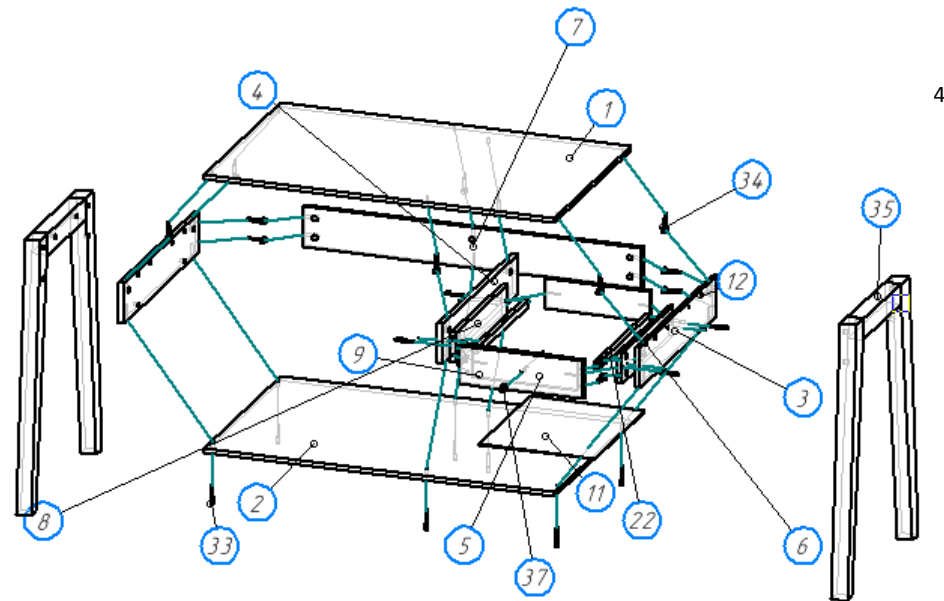
Рис.1 Сборка корпуса
